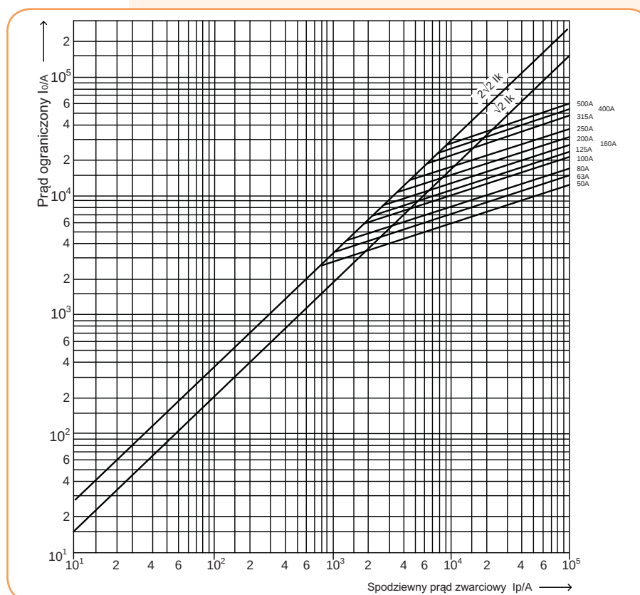
Charakterystyki prądów ograniczonych wkładek topikowych o charakterystyce gG - 1200V - 1XL, 2XL, 3L
