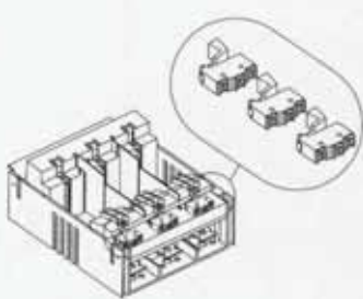
Sposób montażu mikrołączników K-HVL...
