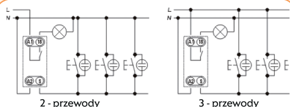
Układ podłączenia
