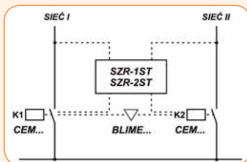
Układ połączeń sterownika do 2 źródeł zasilania
