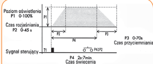
Diagram działania DIM 2
