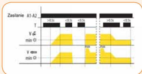
Diagram działania
