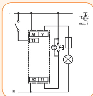
Układ podłączenia
