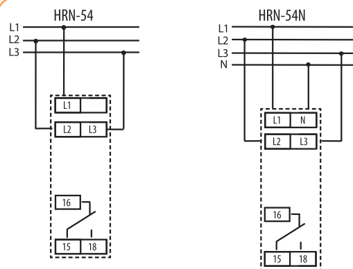
Układy połączeń
