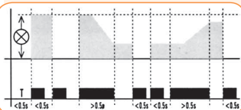
Diagram działania ściemniacza SMR-S
