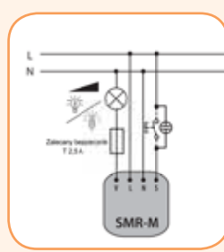
SMR-M schemat podłączenia
