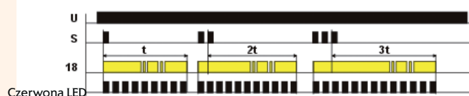
Diagram programowania
