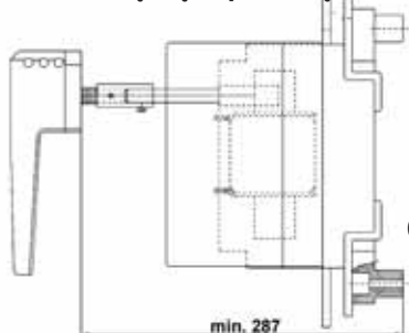
LAF5/R 630 z rączką bezpośrednią
