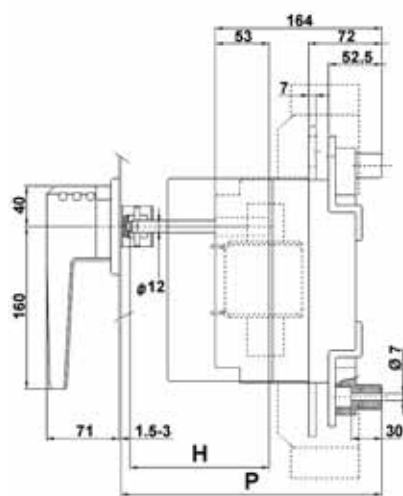
LAF5/R 630 z rączką bezpośrednią
