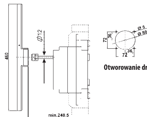
LA5 1250 z rączką bezpośrednią
