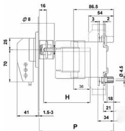
LAF1/R 100 z rączką bezpośrednią
