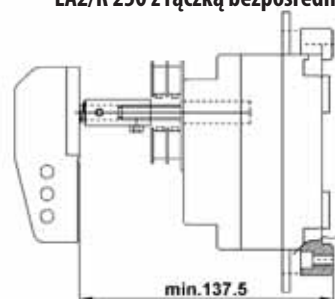
LA2/R 250 z rączką bezpośrednią
