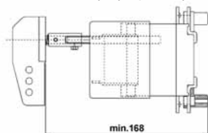
LAF1/R 100 z rączką bezpośrednią
