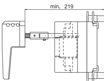
LAF3/R 250 z rączką bezpośrednią
