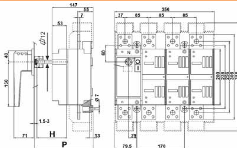
LA5/D 1250 z rączką drzewiową
