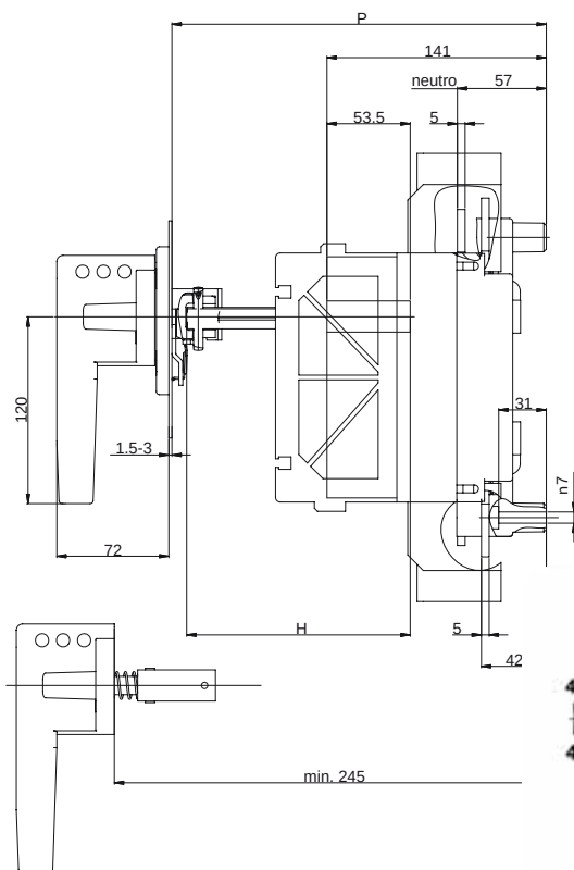
LAF4/R 400 z rączką bezpośrednią
