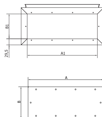
Pokrywa przepustu kablowego
