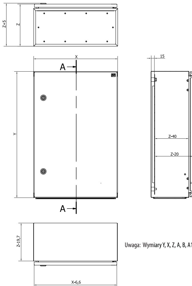
Obudowa kompletna
