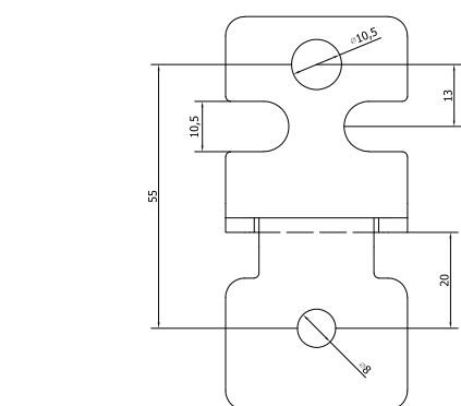
Otwory montażowe w drzwiach pod zamki
