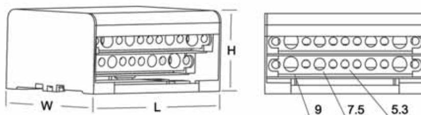
Rysunek wymiarowy
