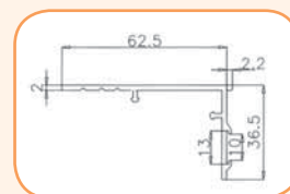
Profil kątowny
