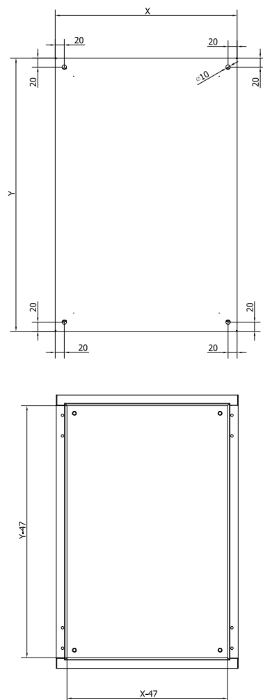
Korpus obudowy
