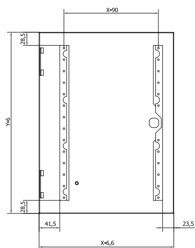
Uchwyt na ścianę
