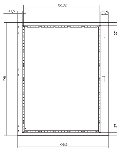
Płyta montażowa
