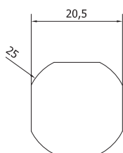
Otwór pod zamek 1 punktowy
