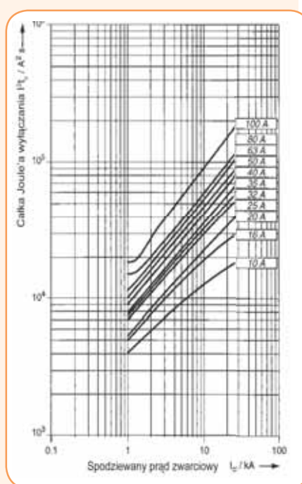
Charakterystyka I²t wyłączników selektywnych ETIMAT S
