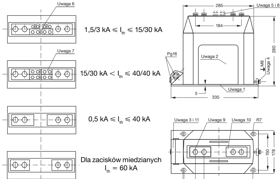
Sposób łączenia zacisków uzwojenia pierwotnego
