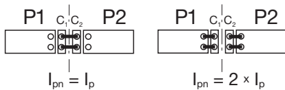
Sposób łączenia zacisków uzwojenia pierwotnego
