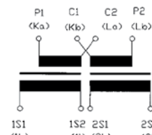
f) Wykonanie przekładnika przełączalnego po stronie pierwotnej z dwoma rdzeniami
