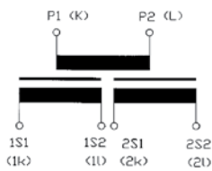
b) Wykonanie z dwoma rdzeniami
