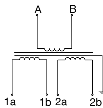
Przekładnik napięciowy jednofazowy, nieziemiany z dwoma uzwojeniami wtórnymi
