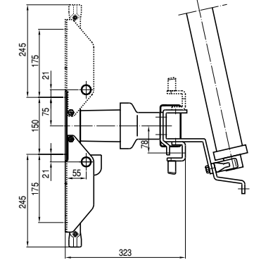
Uziemnik ze zdolnością załączania typu E 24 montowany na podstawie F 24
