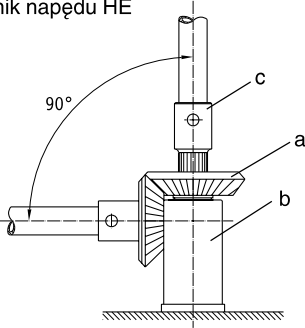
Rys. 24 Przedłużacz wału
